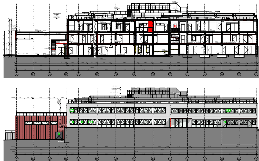
Schnitt A-A, Ansicht Südwest
