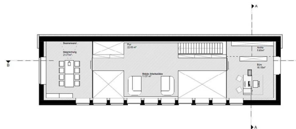
Grundriss Obergeschoss
