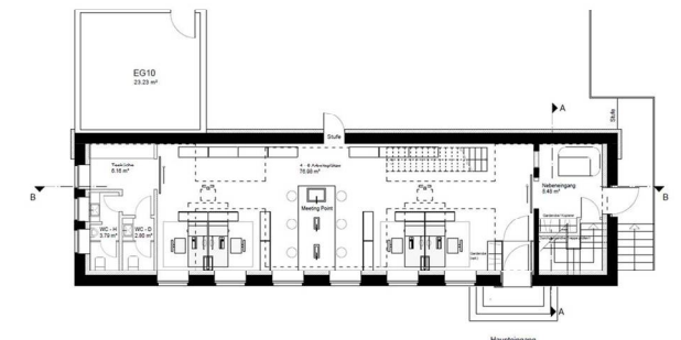
Grundriss Erdgeschoss
