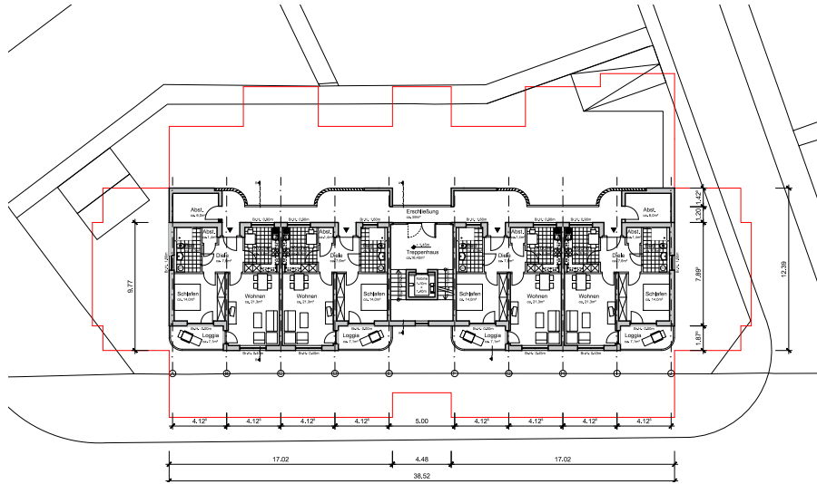
Grundriss Erdgeschoss
