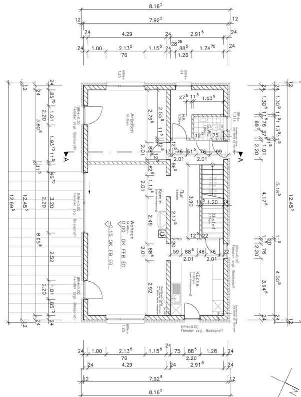
Grundriss EG
