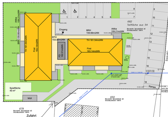
Lageplan
